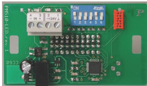
PM510/LED-GN/F Rückansicht
