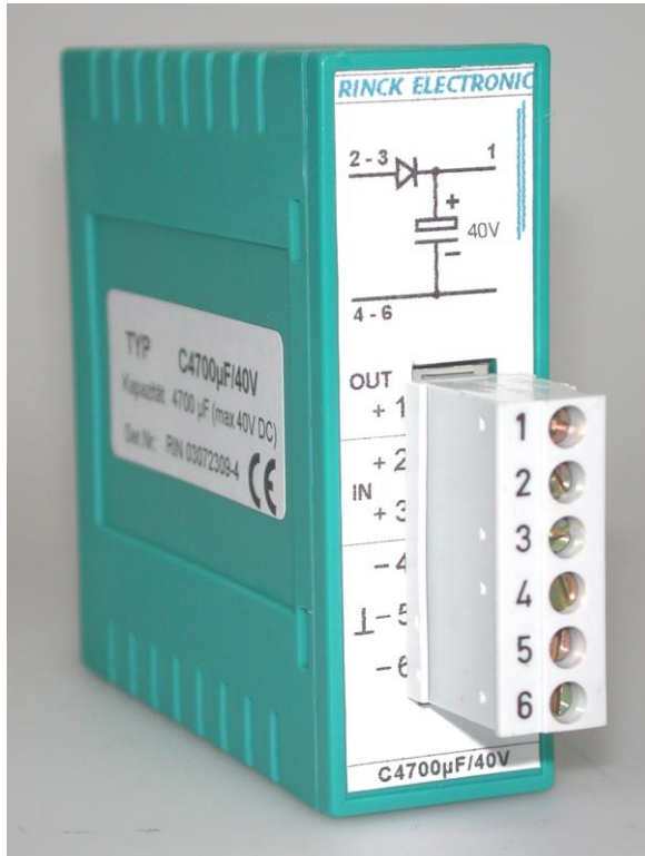
C4700µF/40V
